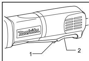
1. Botón de bloqueo 2. Gatillo del interruptor
